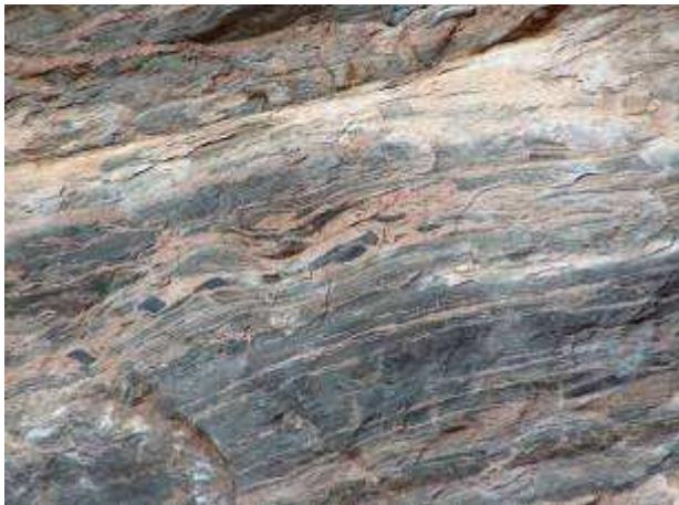
Figures 3.6 : Vues de détail (Fig. 3.5). (a) à gauche, brèche migmatitique et niveaux restitiques à amphiboles . (b) à droite, détail de la texture migmatitique ( x=424427m, y=463957m ).
