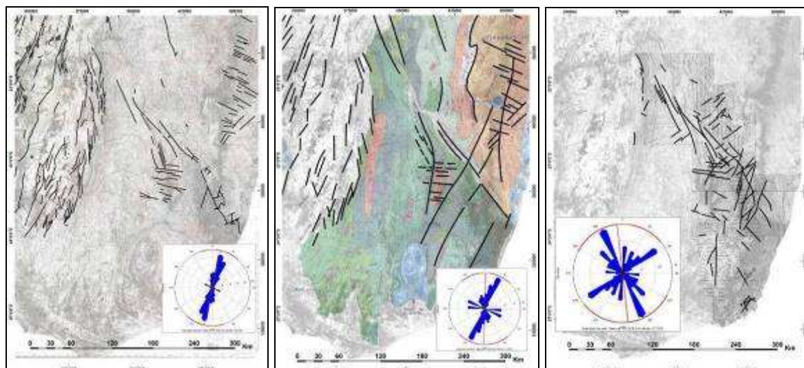
Figures 2.5 : Cartes des fractures de synthèse du \frac{3}{4} sud de Madagascar (sur un fond transparent géologique) et statistique des failles : (a) à gauche carte de synthèse au 1/500000 (Besairie, 1970) (b) au centre synthèse au 1/2000000 (Hottin, 1972) (c) à droite carte de synthèse au 1/2000000 (Bazot, 1976) . Insère sur les cartes, les diagrammes de rose d'orientation des failles (de gauche à droite le nombre de failles analysées : n=440 ; n=136 ; n=95 ). De grandes failles ont été cartographiées sur la carte au 1/2000000 (Hottin, 1972), qui n'existent pas sur la synthèse au 1/500000 (Besairie, 1970). Sur la carte de Bazot (c), la zone de failles cartographiées n'est pas la même que pour Besairie et Hottin (a et b). Les directions qui ressortent sont également différentes. On observe également que au Sud de la latitude 24^{\circ} S, très peu de fractures (voire aucune) n'ont été cartographiées par ces trois auteurs.
