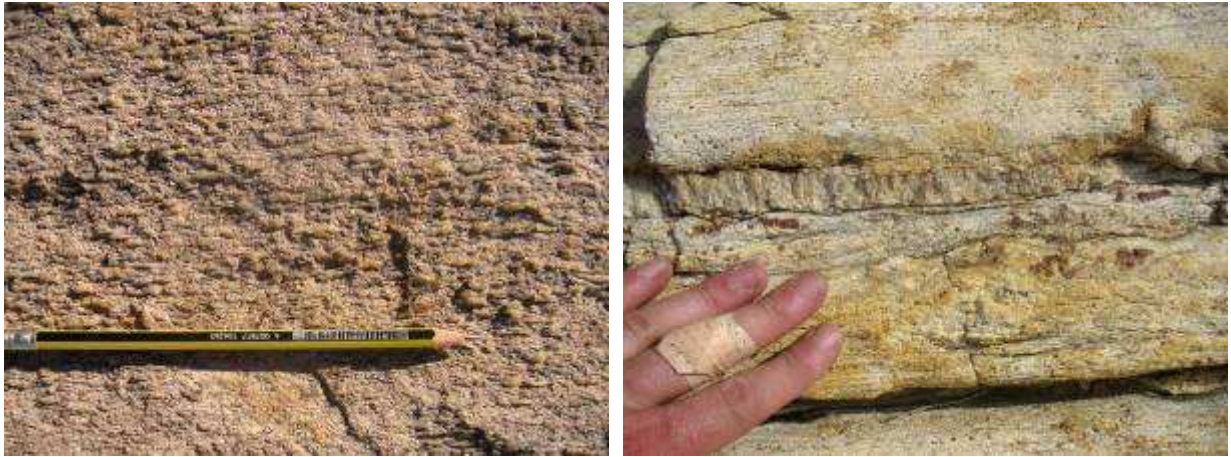
Figures 3.23 : (a) à gauche, détail de la texture de la roche, cristaux de quartz étirés (plan horizontal, x=380098m , y=426163m ). (b) à droite, ruban de quartz étiré sur 10 à 20 cm (plan horizontal, x=392171m , y=393725m ).
