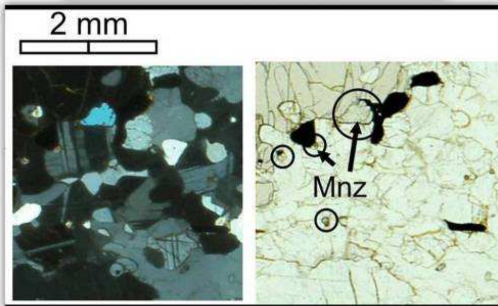
Figures 8. 12 : lame de gneiss alumineux à Grenat Biotite et rares magnétites, riche en monazites en LPNA et détail en LPNA et LPA (monazites de plus de 700 microns). ZC de Beraketa.
