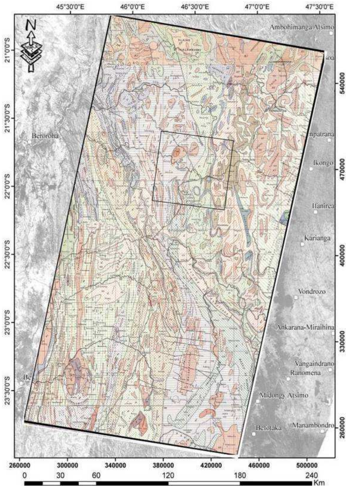
Figure 4.12 : Carte géologique de la région, échelle 1/500000 (Bésairie, 1970).
