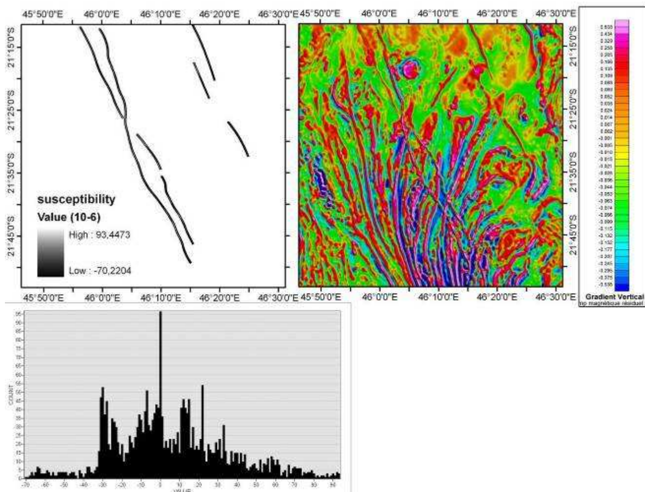
Figure 9.17 : En haut : (a) à gauche, Anomalies linéaires , sécantes sur les trajectoires de foliations. (b) à droite, composante verticale du champ magnétique résiduel , région Nord (Ihosi). (c) En bas, histogramme de distribution des valeurs de susceptibilité des linéaments (valeur en abscisse de -70 à 93 \cdot 10^{-6} SI ; moyenne autour de 10 \cdot 10^{-6} SI).
