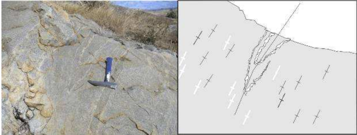
Figures 3.27 : (a) à gauche, gneiss migmatitiques à amphibole et plis ptygmatisés compatibles avec un raccourcissement Est-Ouest. (b) à droite, dessin interprétatif : le plan axial est N 0° peu penté vers l'Est (x=411247m, y= 461148m). Plan vertical.
