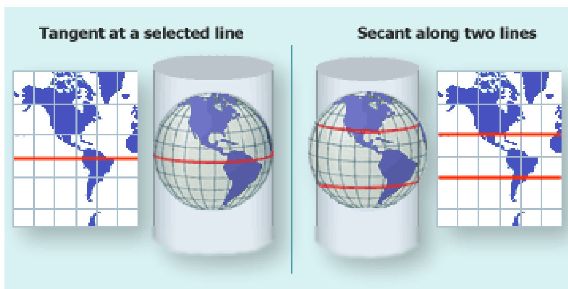
Figure 1.9 : Projection cylindrique : tangente (à gauche) et sécante (à droite), (http://nte-serveur.univ-lyon1.fr/) .
