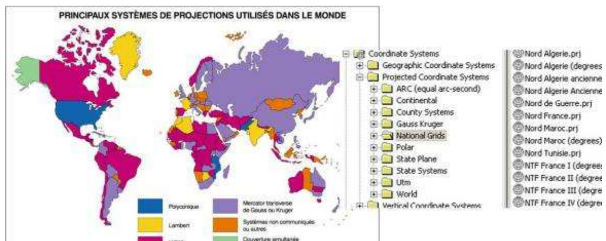
Figure 1.7 : (a) à gauche, carte des Principaux systèmes de projections utilisés dans le monde ( http://hydrasa.labo.univ-poitiers.fr/jbodin/recherche.htm ); (b) à droite, exemples de systèmes de projections utilisés par arcGIS.
