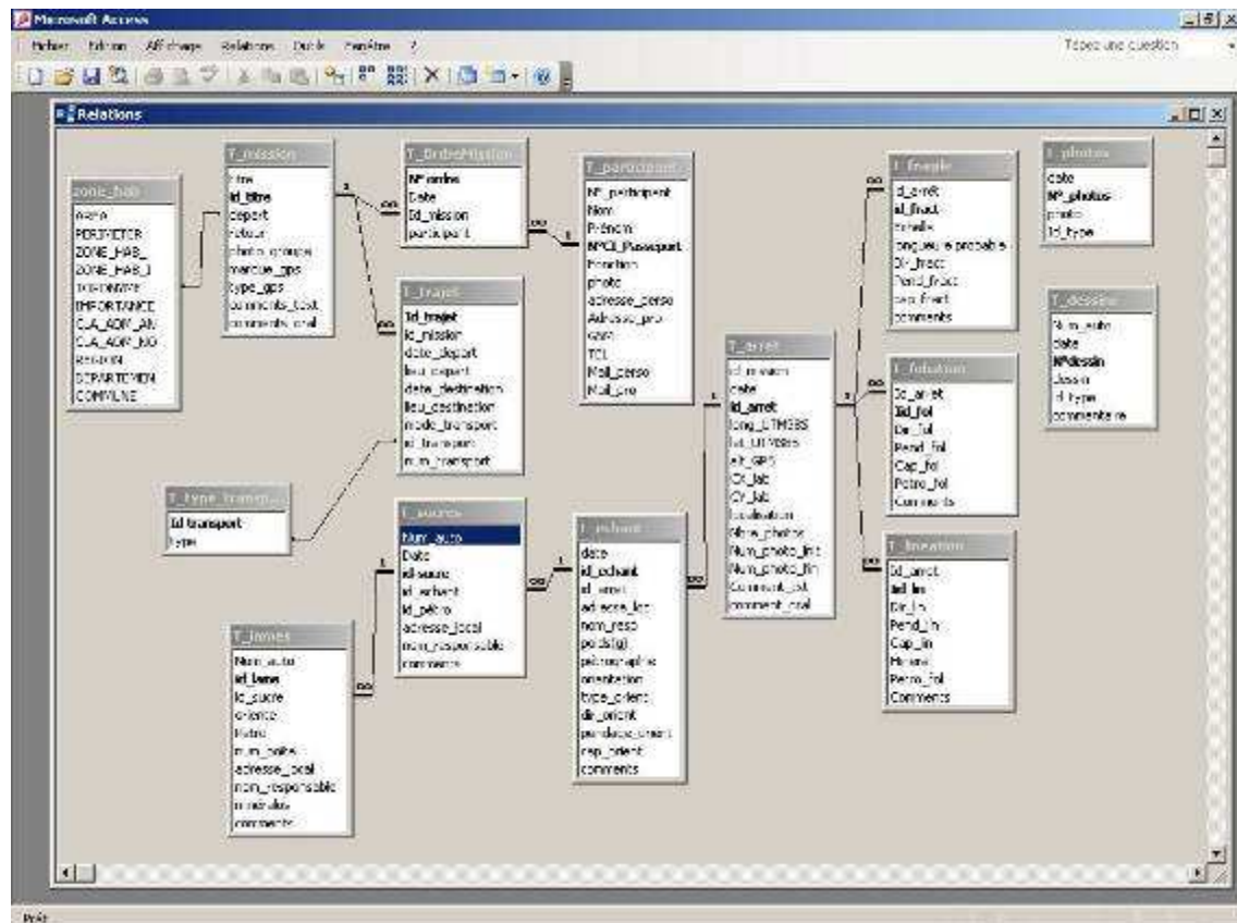
Figure 1.15 : Relations entre les tables des données de terrain (Microsoft Access 2003).
