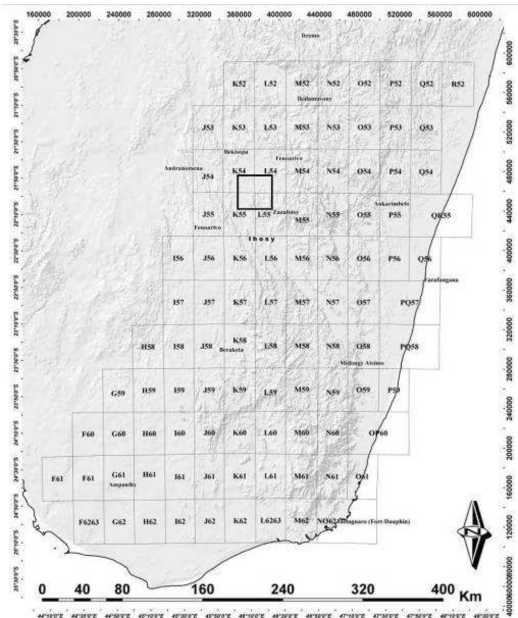
Figure 3.1: Limite des coupures de cartes à l'échelle 1/100 000 ème utilisées, les Figures 3.3 sont localisées par le carré noir.
