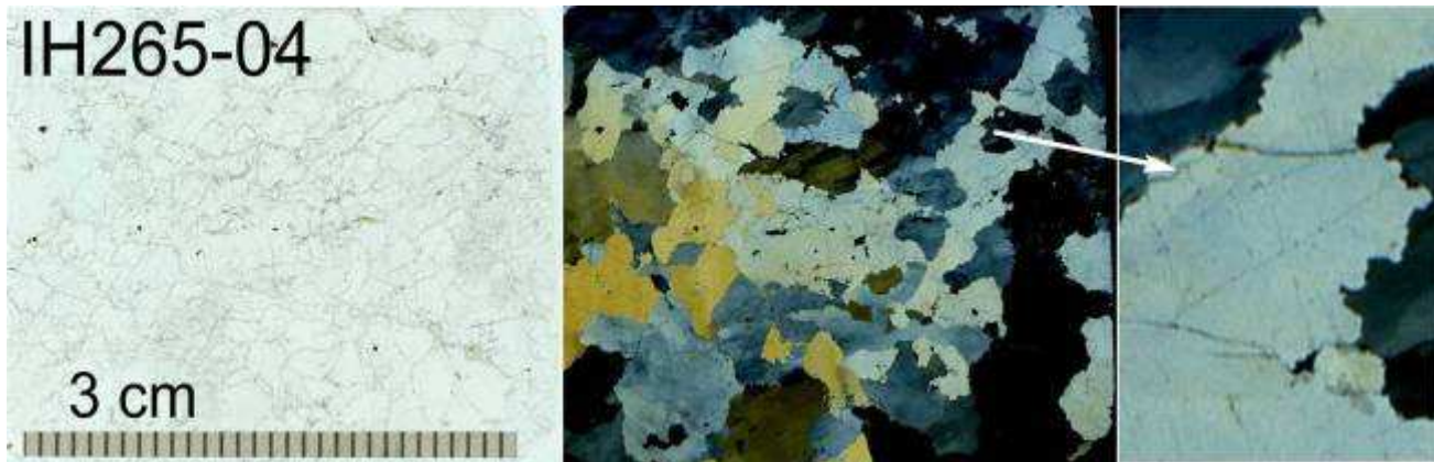
Figures 3.8 : Lame mince de quartzite (a) à gauche, en LPA et (b) à droite, en LPNA . La quartzite est très pure et montre des grains de grandes tailles (plurimillimétriques) avec des limites très digitées (x=418509m, y= 464274m).
