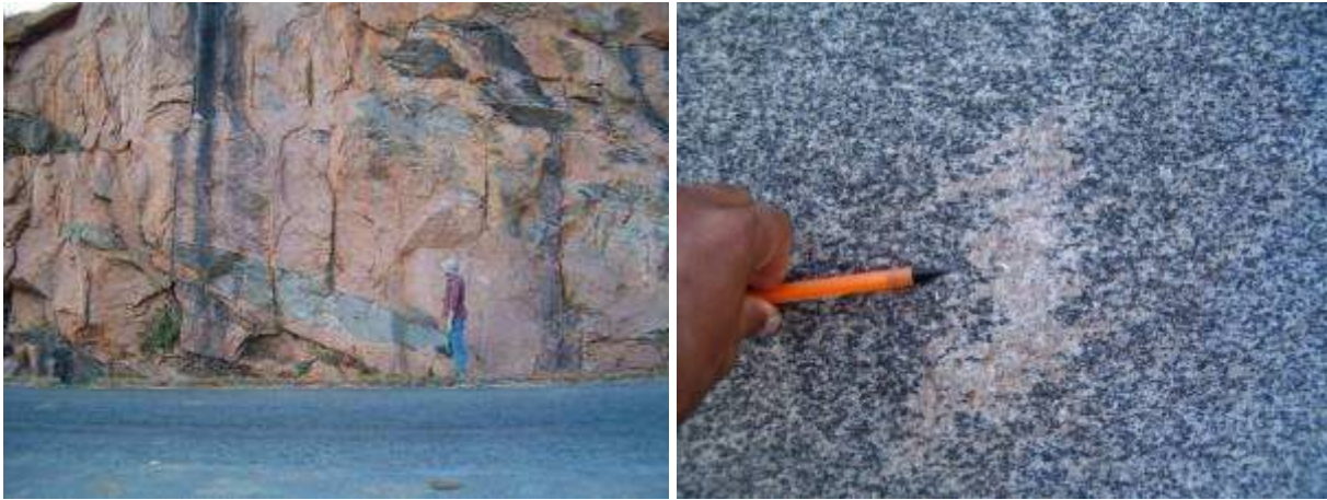
Figures 3.3 : (a) à gauche, large corps granitique avec enclave de gneiss à amphibole montrant une forte fabrique et des plis compatibles avec un aplatissement vertical ( x=444339m , y= 476359m ). (b) à droite, plan horizontal, derniers magmas à cristalliser dans une syénite ( x=434504 m , y= 470483m ).
