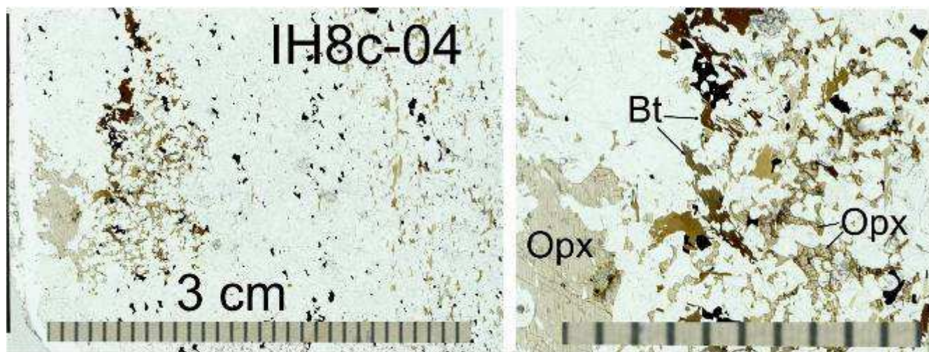
Figure 3.16 : (a) à gauche, lame mince de charnockite en LPNA : dans le plan S1 les orthopyroxènes et les biotites sont visibles (plan vertical), aux dépens des biotites, les orthopyroxènes se développent également dans les deux plans S1 et S2. La charnockitisation est moins importante et parfois absente dans le plan S1 (lit à biotite non perturbée dans la partie droite de l'image). (b) Détail de la texture , l'orthopyroxène peut atteindre 4 mm de long et la biotite est en symplectique ou complètement consommée aux dépens de l'orthopyroxène ( x=395156m , y=455254m ).
