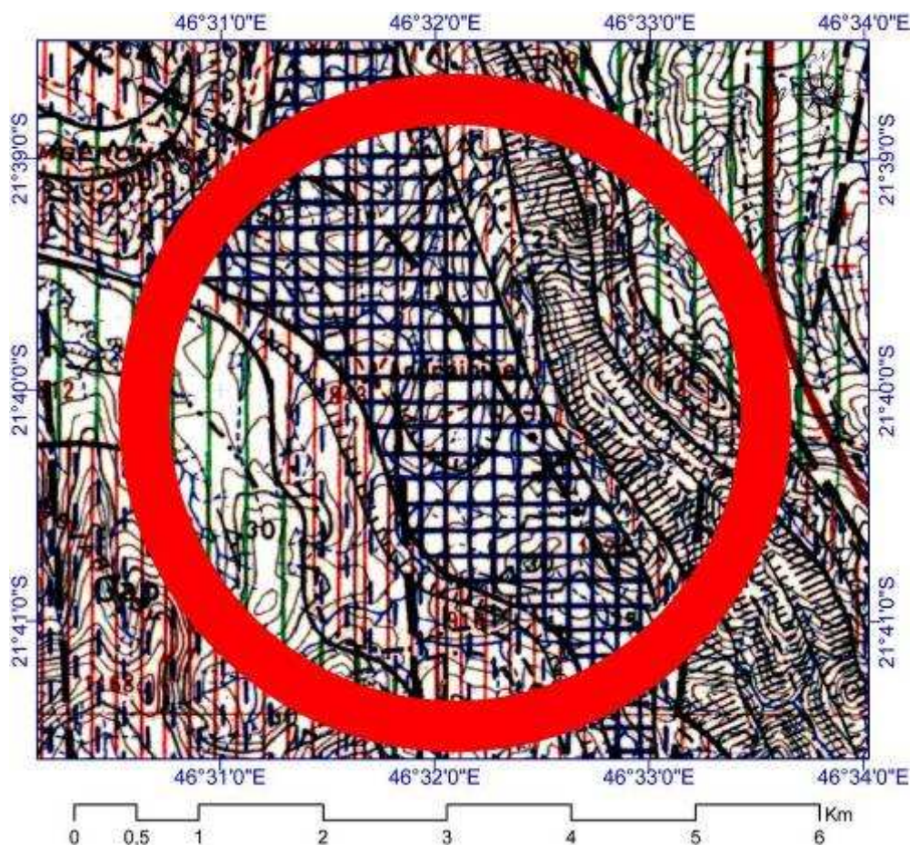
Figure 4.19 : Région de Fenarivo (Nord – Ouest d’Ankaramena : relation « bull-eyes », ZC, et dykes (a) page précédente, sur une carte de champ magnétique résiduel H' , avec localisation d’une caldeira (cercle rouge) sur la carte géologique 1/100 000, feuille M54. Les « bull-eyes » sont associés principalement à de grands dykes kilométriques, ainsi qu’à leur intersection avec (i) d’autres dykes (cas BE1), (ii) des directions de foliations majeures (cas BE2), (iii) l’intersection avec la ZC de Zazafotsy (cas BE3), et (iv) un réseau d’anomalies ponctuelles négatives (cas BE4). Deux ZC (limites en lignes blanches) sont visibles sur cette image : la ZC de Morarano (à l’Ouest) et celle de Zazafotsy (à l’Est) ;
