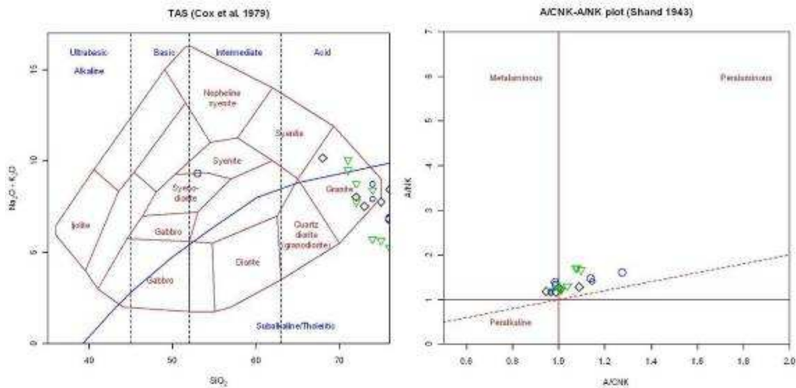
Figure 8.13 : (a) à gauche, diagramme de \text{Na}_2\text{O}+\text{K}_2\text{O} versus \text{SiO}_2 . (b) à droite, diagramme de Shand, (1843) . L'ensemble des roches sont à caractère granitique avec un trend montrant des valeurs relativement fortes \text{Na}_2\text{O}+\text{K}_2\text{O} , une roche montre des teneurs en \text{SiO}_2 compatibles avec une composition syénitique.
